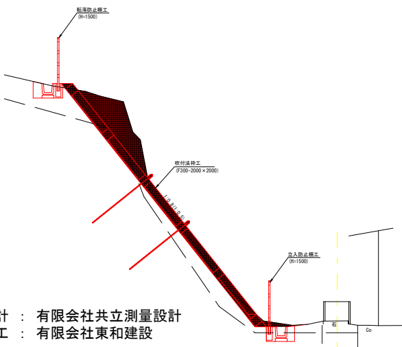
標準断面図
