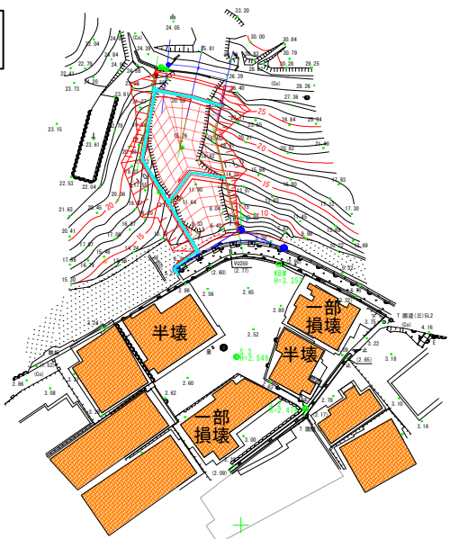
平面図
