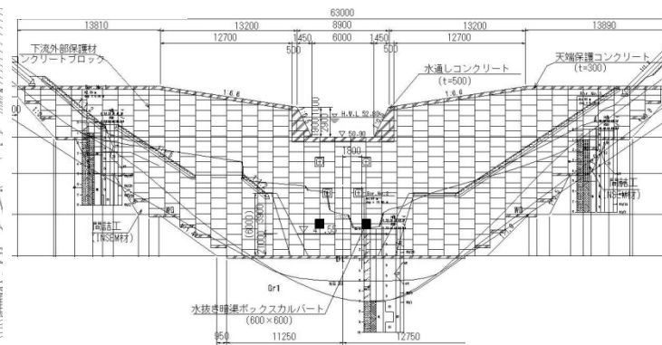
【正面図(本堤工)】
