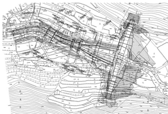
【平面図(事業全体)】
