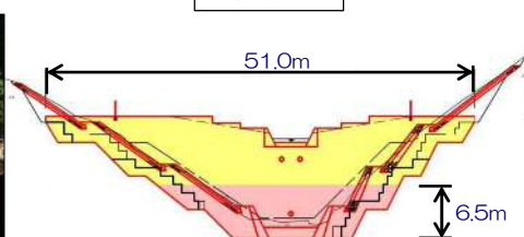
堰堤一般図
