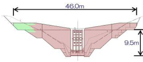
堰堤一般図
