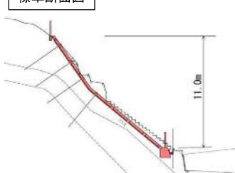
標準断面図
