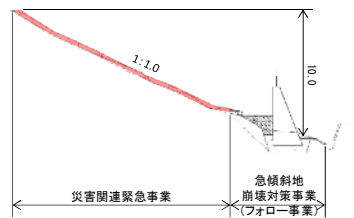
標準断面図
