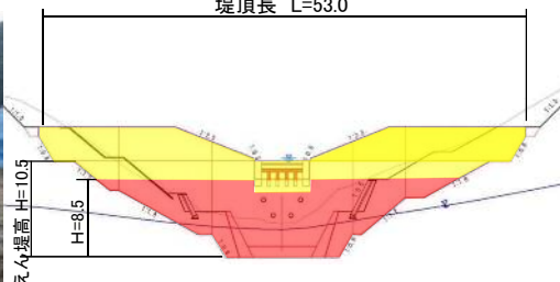
堰堤一般図
