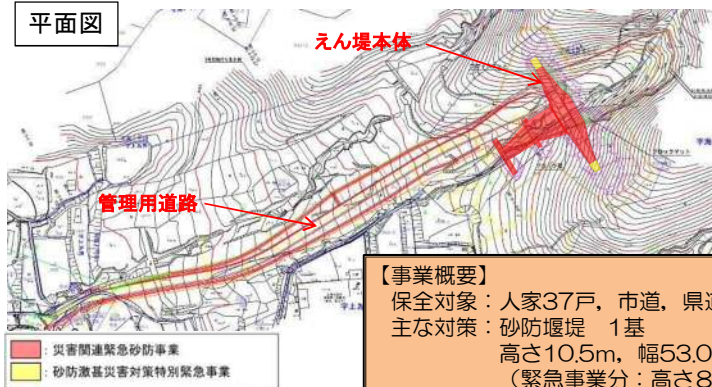
堰堤一般図
