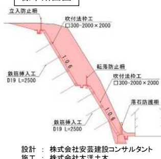
標準断面図
