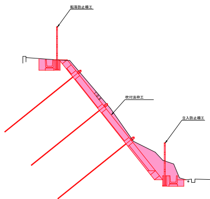
標準断面図
