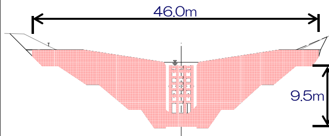
堰堤一般図
