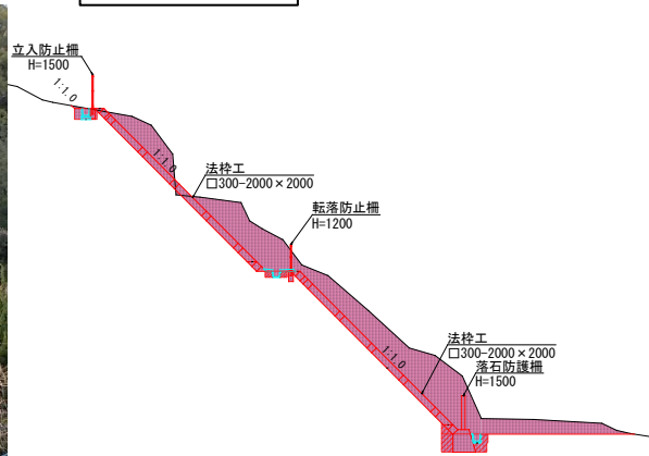
標準断面図
