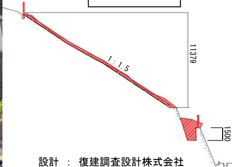
標準断面図
