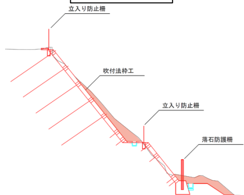
標準断面図
