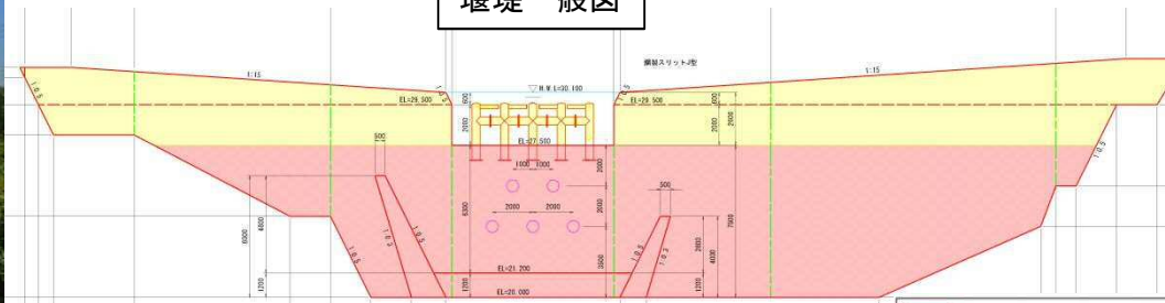
堰堤一般図
