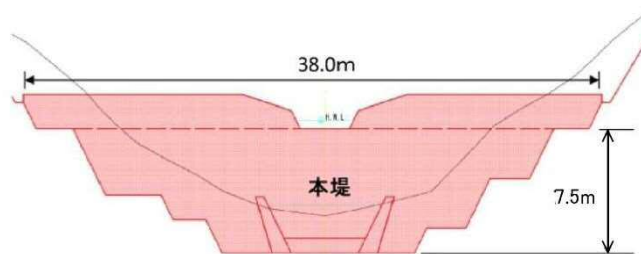
堰堤一般図
