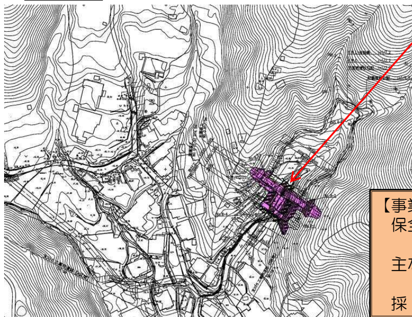
堰堤一般図
