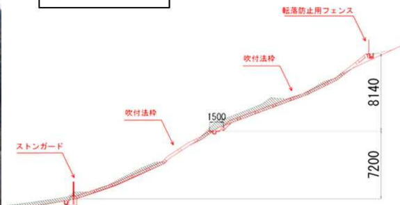
標準断面図
