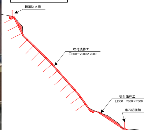
標準断面図
