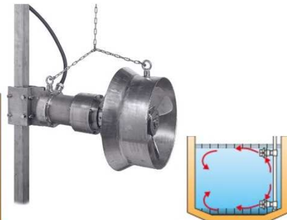
Horizontal stirrer
