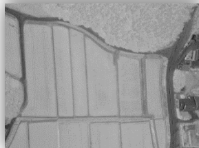
NDVI画像
