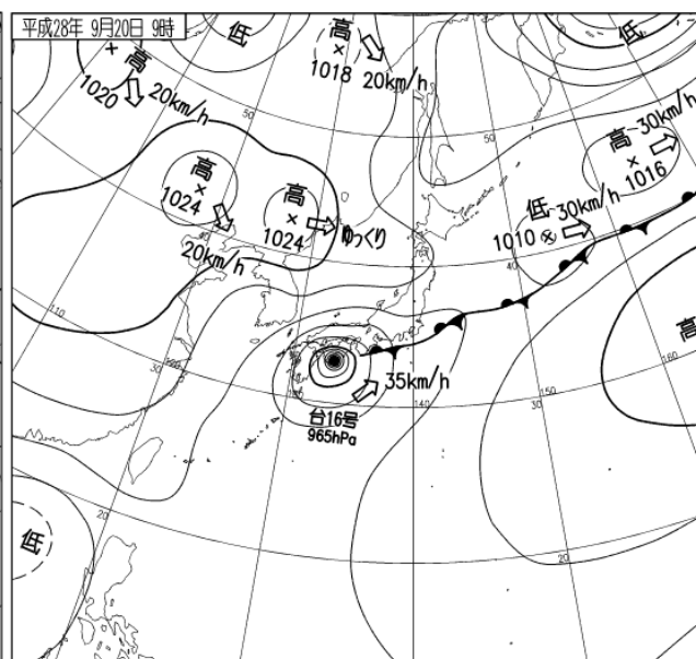
平成 28 年 9 月 20 日 09 時 地上天気図
