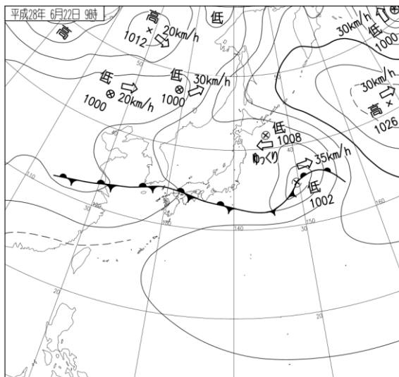
平成 28 年 6 月 22 日 09 時 地上天気図
