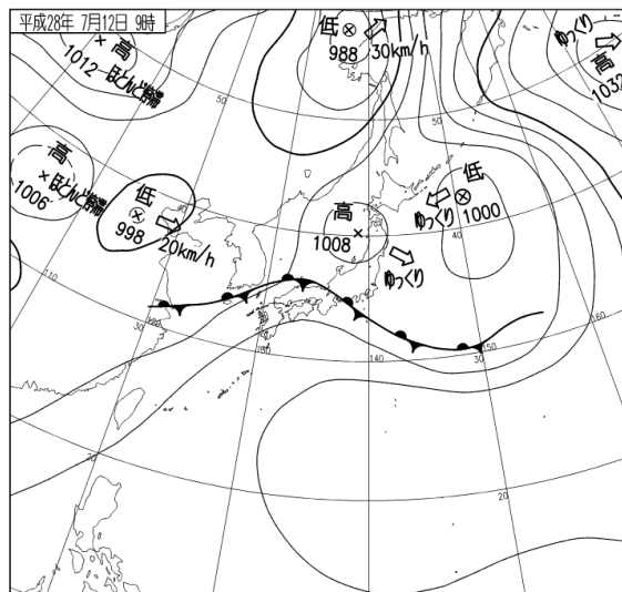
平成 28 年 7 月 12 日 09 時 地上天気図
