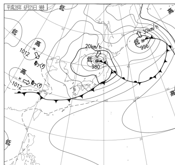
平成 28 年 6 月 25 日 09 時 地上天気図
