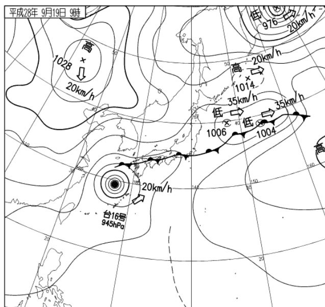
平成 28 年 9 月 19 日 09 時 地上天気図
