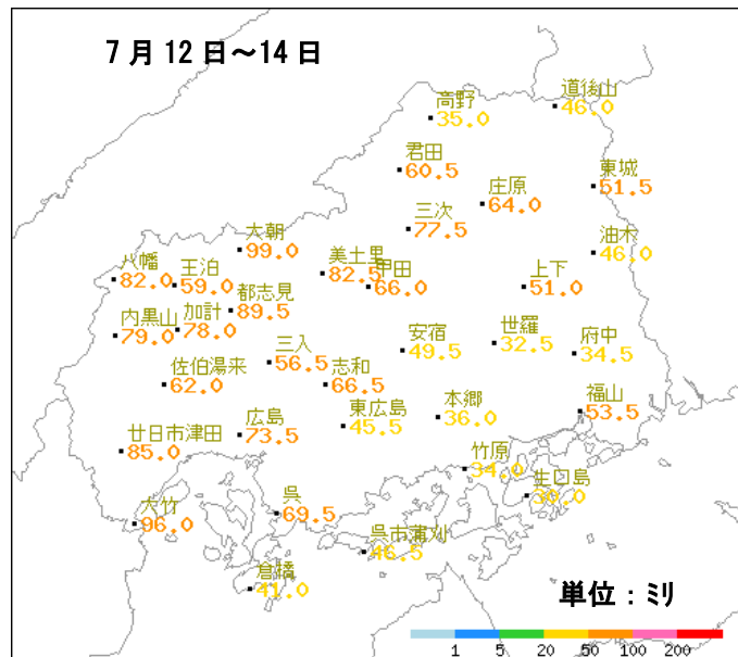
アメダス地点の降水量分布図
