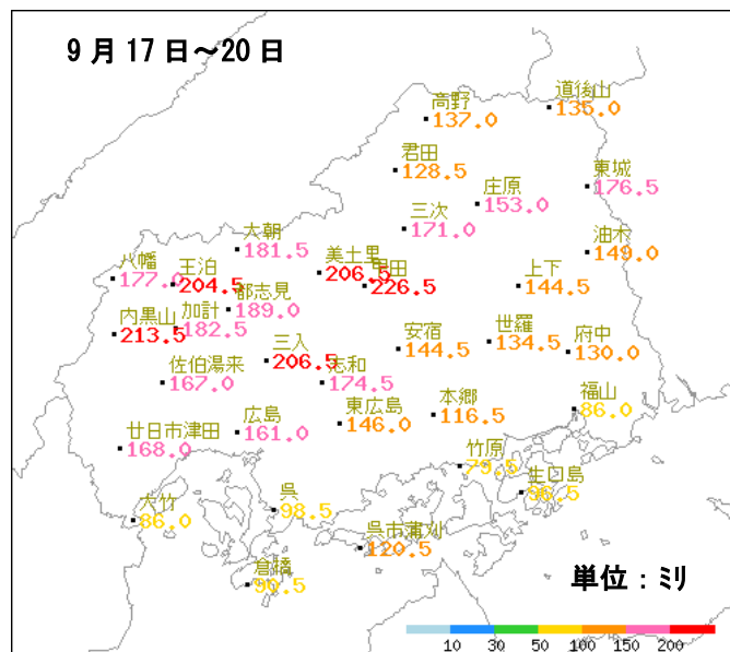
アメダス地点の降水量分布図 平成 28 年 9 月 17 日～20 日
