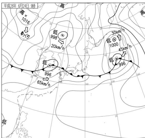
平成 28 年 6 月 24 日 09 時 地上天気図
