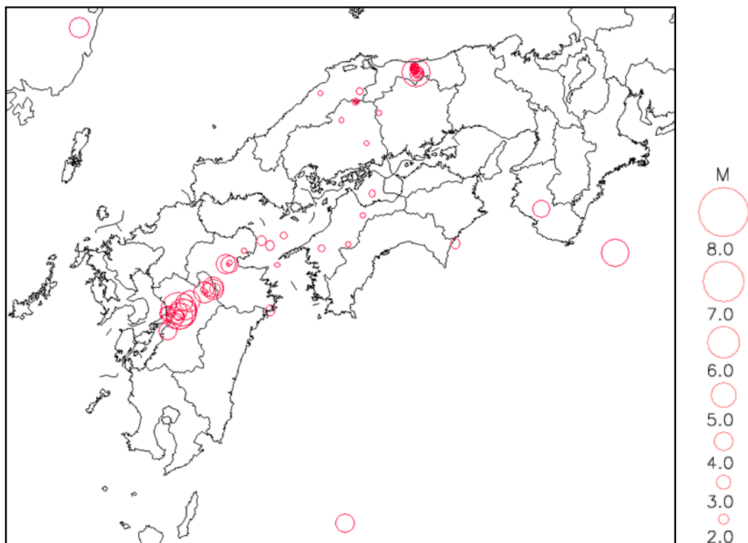
2016（平成28）年に広島県内で震度1以上を観測した地震の震央分布図
