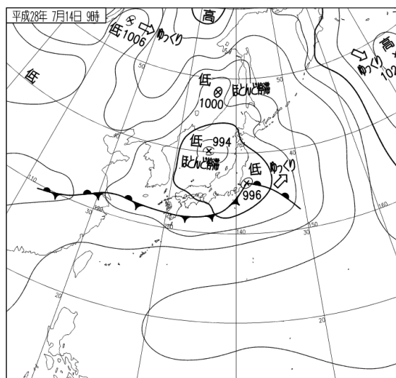
平成 28 年 7 月 14 日 09 時 地上天気図
