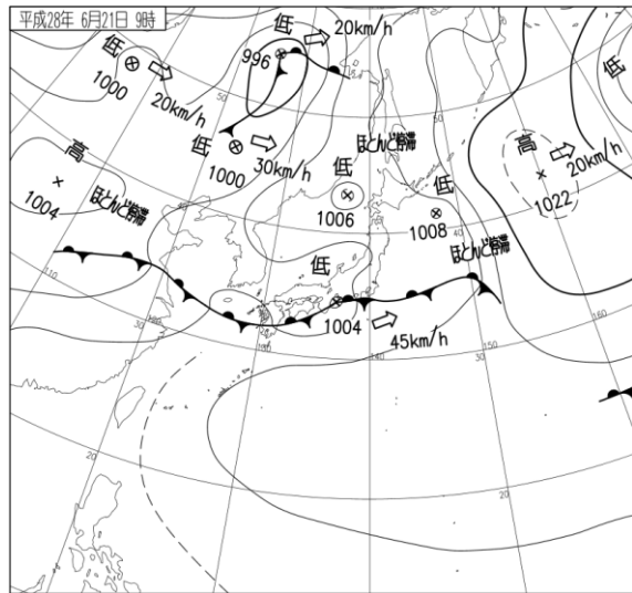
平成 28 年 6 月 21 日 09 時 地上天気図
