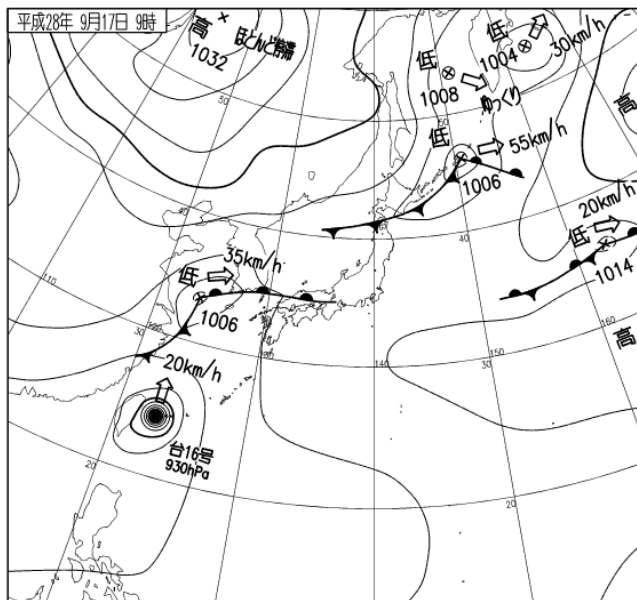
平成 28 年 9 月 17 日 09 時 地上天気図
