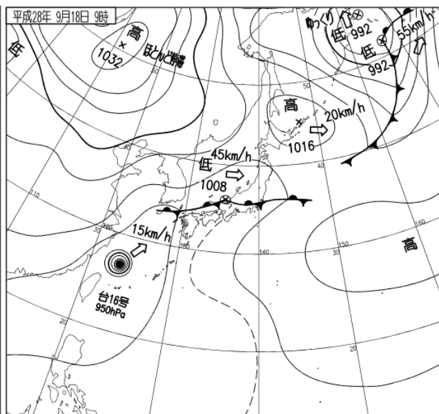
平成 28 年 9 月 18 日 09 時 地上天気図
