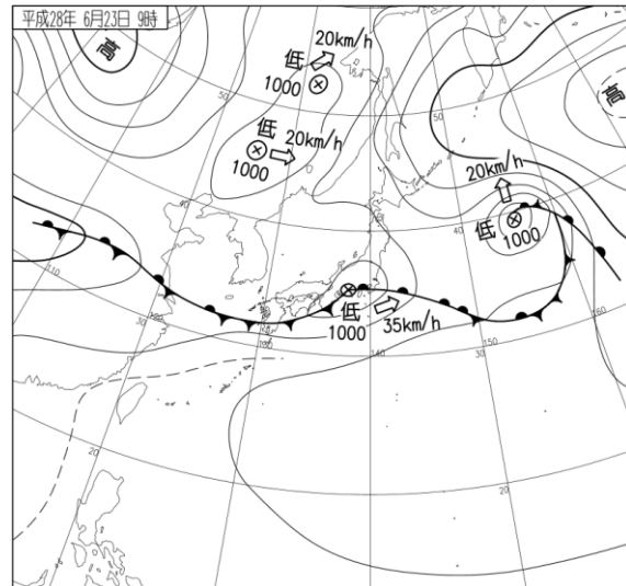
平成 28 年 6 月 23 日 09 時 地上天気図
