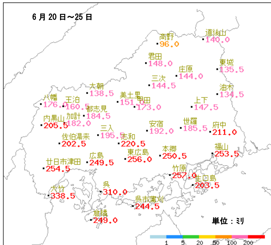
アメダス地点の降水量分布図
