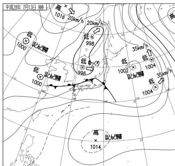
平成 28 年 7 月 13 日 09 時 地上天気図
