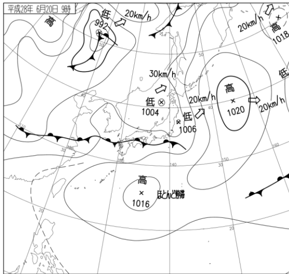
平成 28 年 6 月 20 日 09 時 地上天気図
