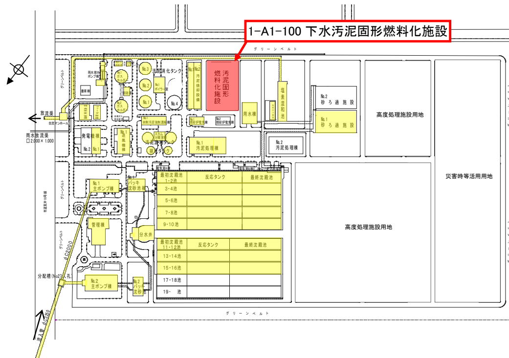
芦田川浄化センター平面図
