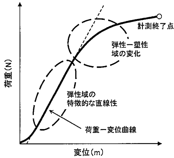
図 3. 荷重-変位曲線の適切な事例
