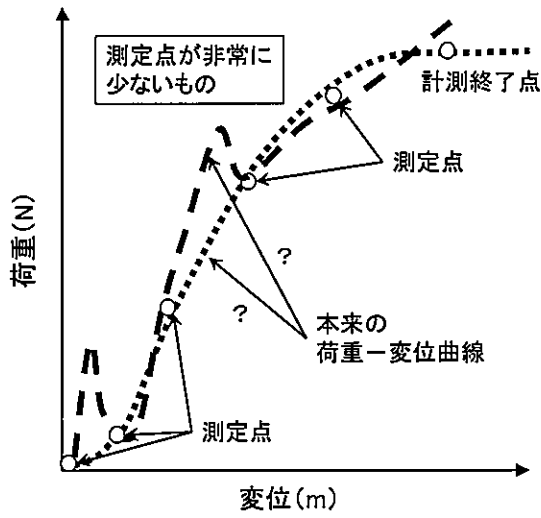
図 4. 荷重-変位曲線の不適切な事例
