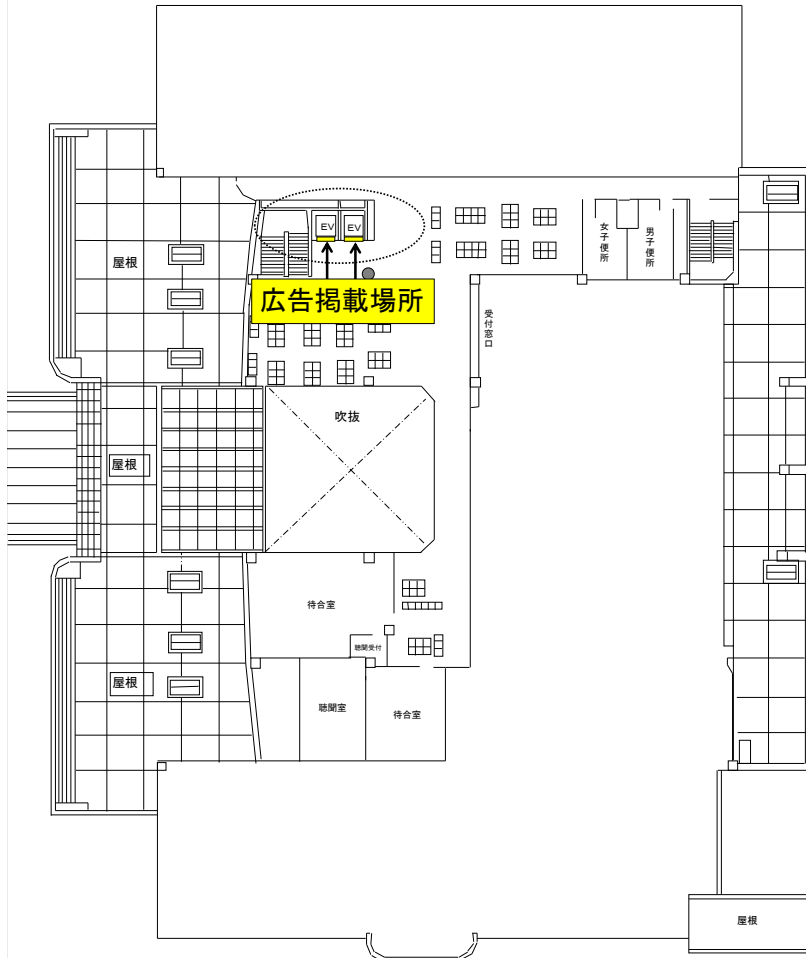
3階平面図
