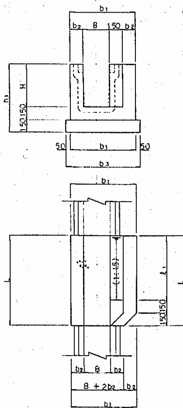
【小動物脱出側溝構造図】
