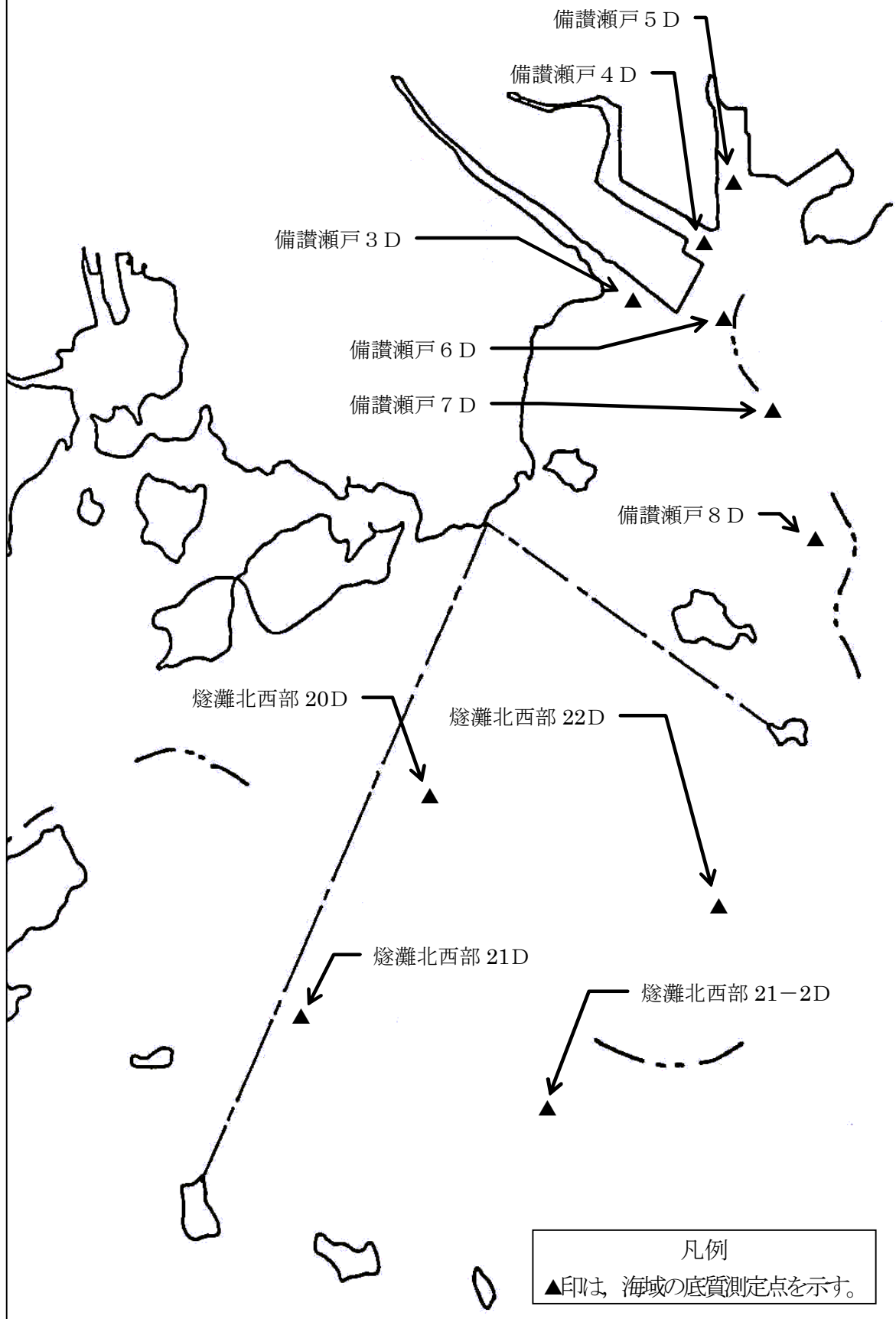
底質調査地点配置図（４）
