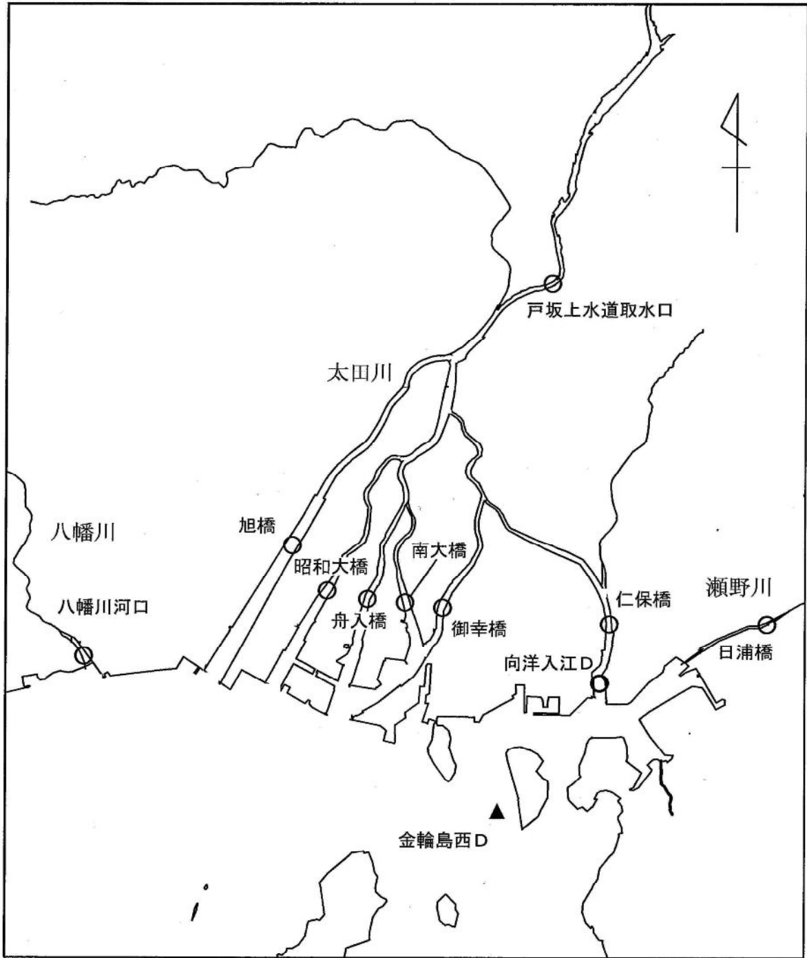
底質調査測定点配置図（1）
