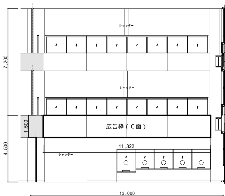
立面図
