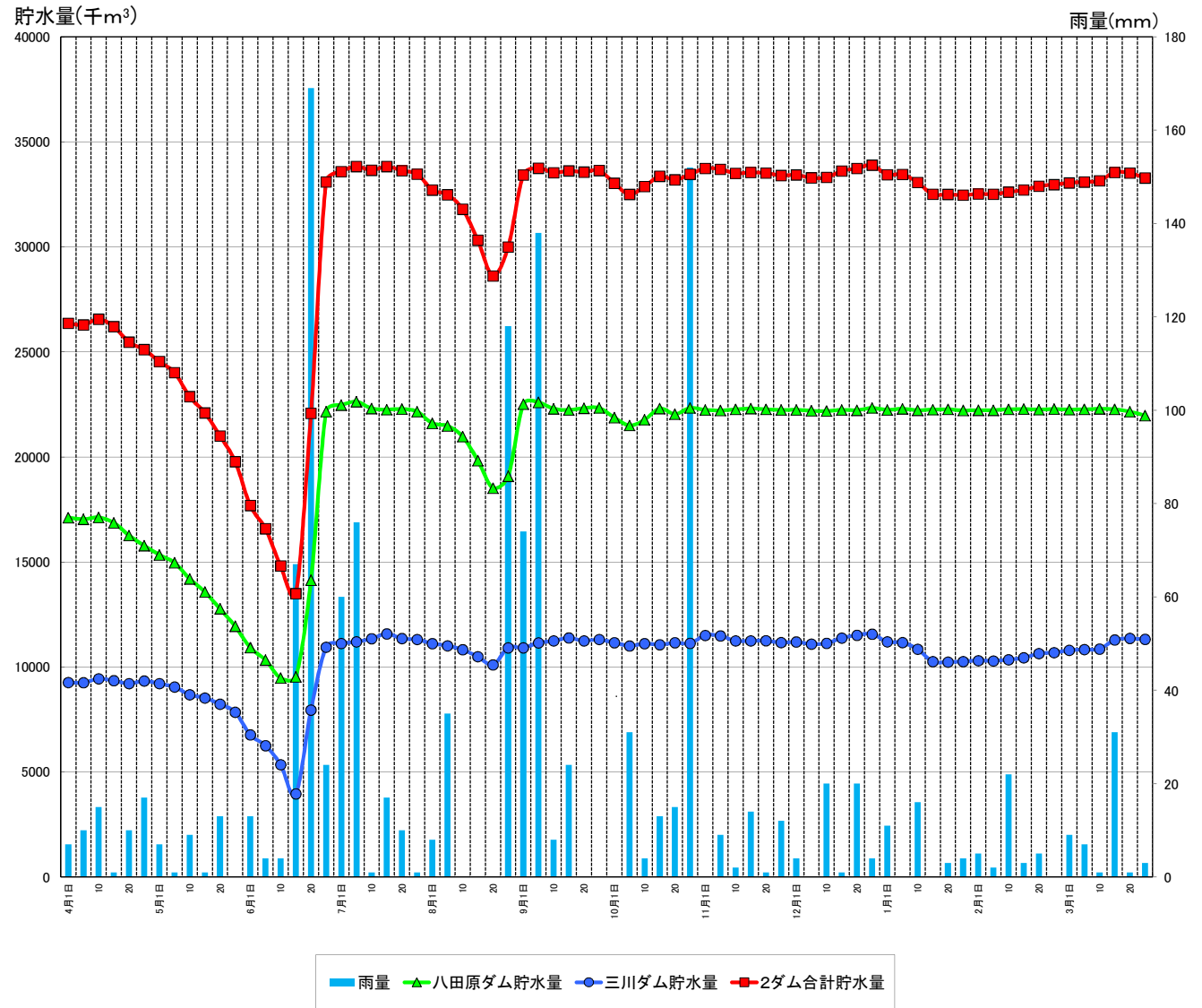
八田原ダム、三川ダムの貯水状況グラフ(H25年度)
