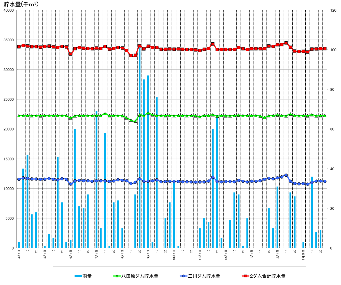
八田原ダム、三川ダムの貯水状況グラフ(H27年度)
