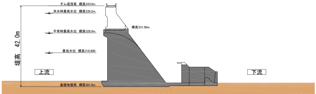
堤体断面図 (ダムの中央部を右岸から見た図)
