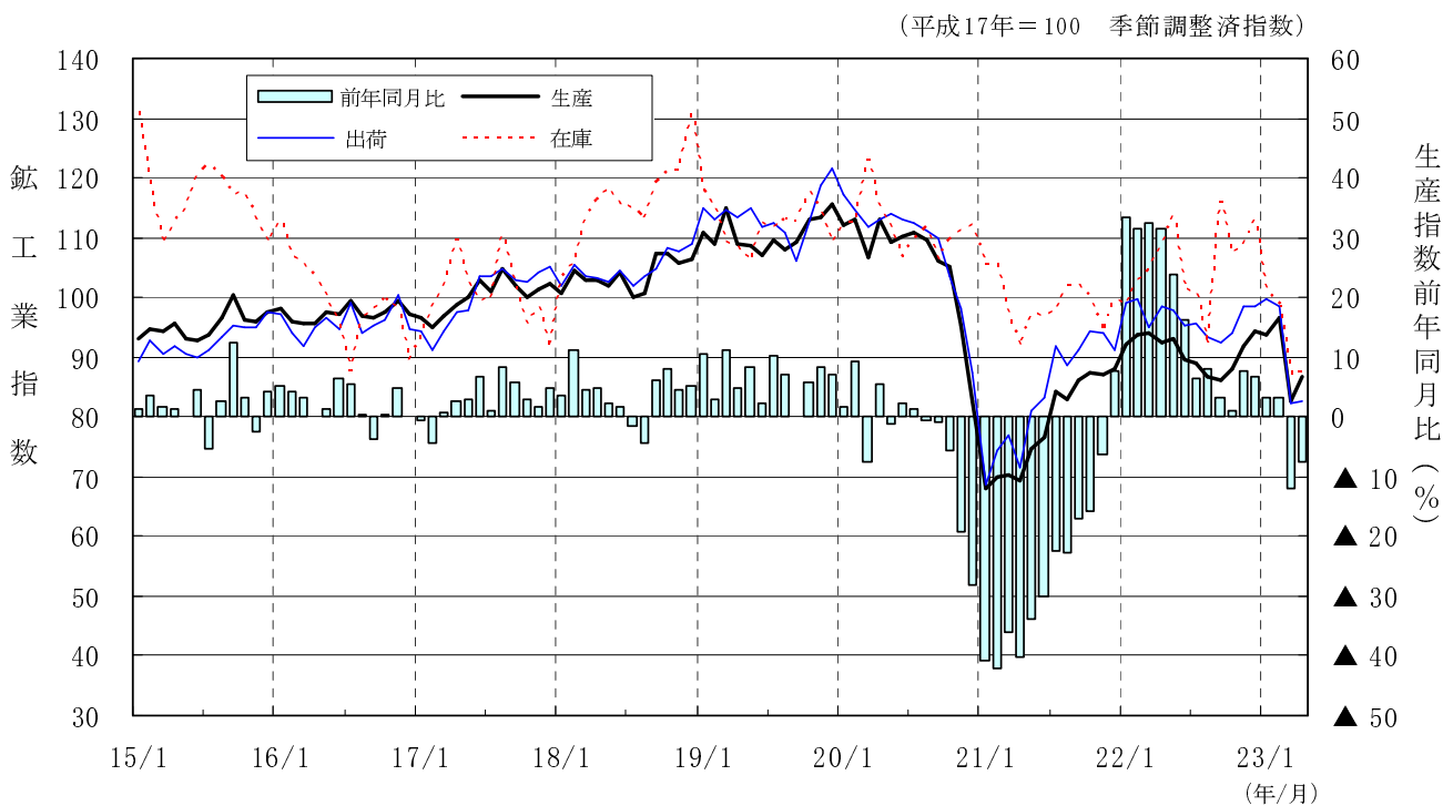
広島県鋳工業指数の推移 (平成 15 年 1 月～平成 23 年 4 月)
