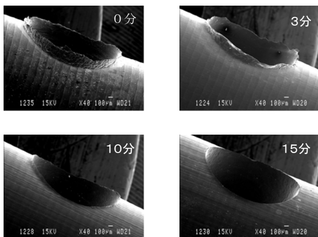
写真1 バリ除去の様子 (SUS304)
