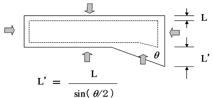
図1 バリ取りの機構
