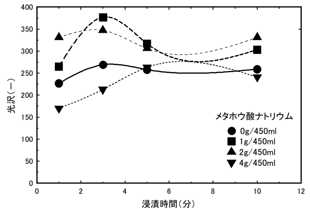
図 3 アルミニウム合金の浸漬時間と光沢の関係 (NaOH 0.14%, A 成分 10%, B 成分 0.05%, 70℃)
