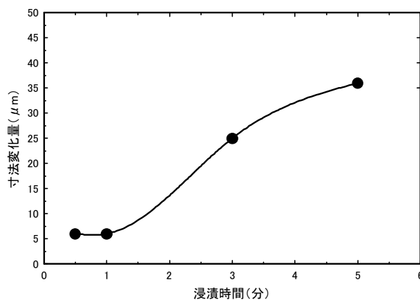
図10 アルミニウム合金の浸漬時間と寸法変化量の関係 (リン酸, C成分, 110~120°C)
