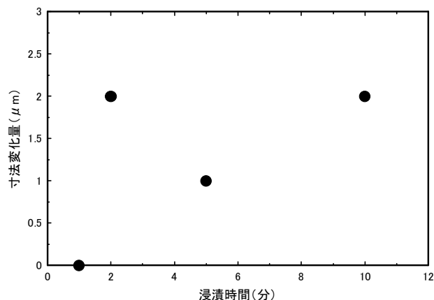
図9 アルミニウム合金の浸漬時間と寸法変化量の関係
