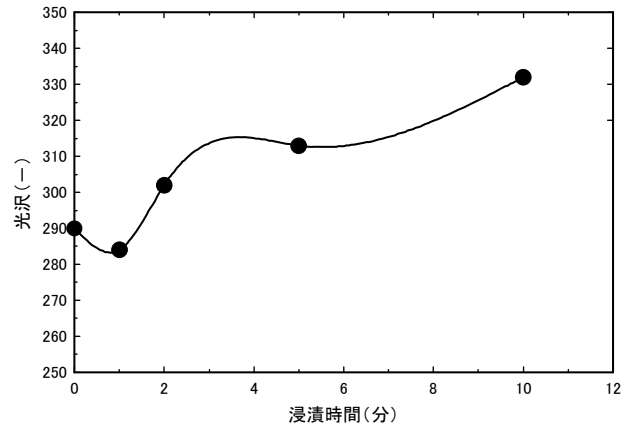
図 2 アルミニウム合金の浸漬時間と光沢の関係 (NaOH 0.2%, A 成分 10%, B 成分 0.1%, 70℃)
