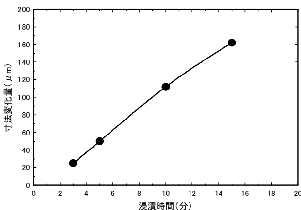
図11 鉄鋼の浸漬時間と寸法変化量の関係 (過酸化水素, 酸性フッ化アンモニウム, D, E成分, 25~35°C)
