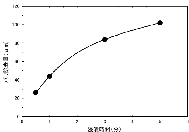
図8 アルミニウム合金の浸漬時間とバリ取り量の関係 (リン酸, C成分, 110~120°C)
