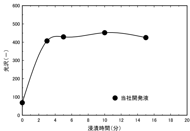
図 5 鉄鋼の浸漬時間と光沢の関係 (25~35°C)
