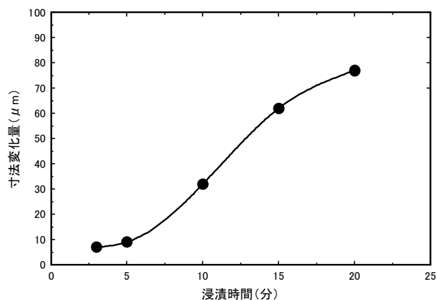
図 1 2 SUS304 の浸漬時間と寸法変化量の関係 (塩酸, 硝酸, リン酸, F, G 成分, 90~95°C)
