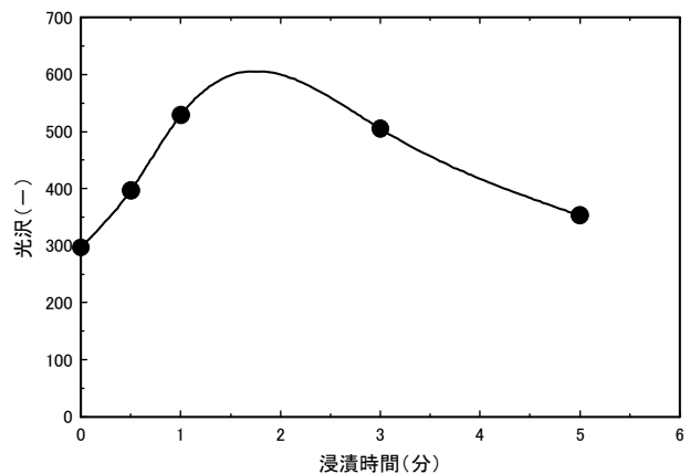
図 4 アルミニウム合金の浸漬時間と光沢の関係 (リン酸, C 成分, 110~120℃)
