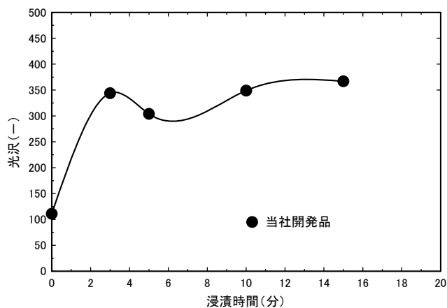
図 6 SUS304 の浸漬時間と光沢の関係 (90~95°C)
