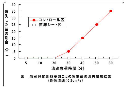
図4-B 苗床シートによる流失防止効果
